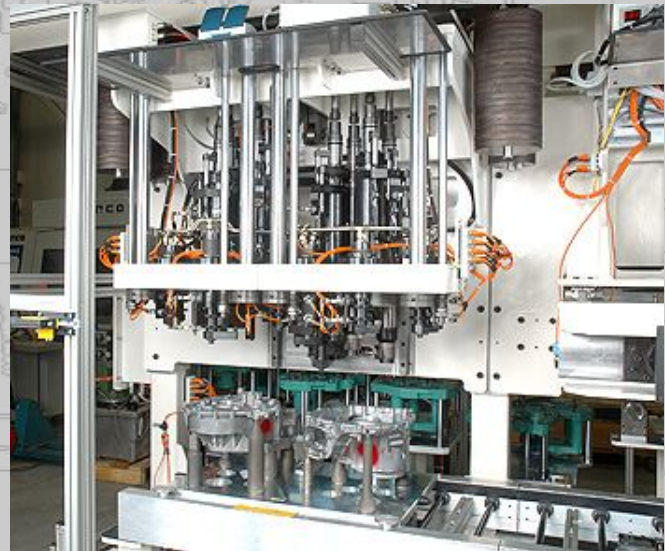
Statisches Vermessen der beiden Getriebegehäusehälften unter Last
